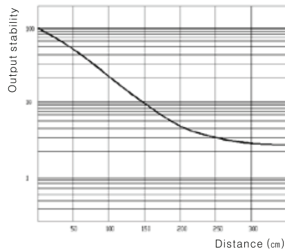
Distance vs Output stability 距離相對於輸出穩定度
