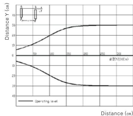
Parallel deviation (Vertical) 平行的偏向 (垂直的)
