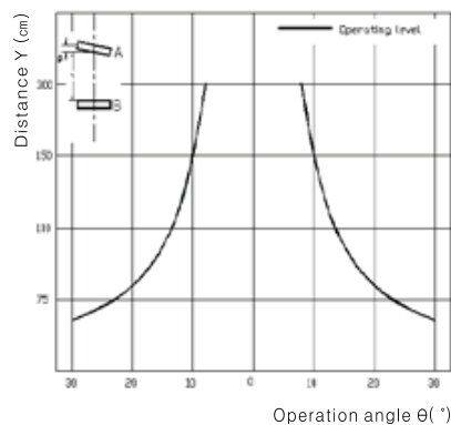
Angular deviation 尖角的偏向
